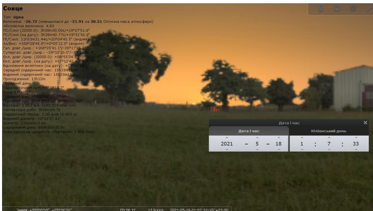
Рис. 1. Скріншот Stellarium. Місце спостереження: широта 70^{\circ} 0' 0.00'' на північ, довгота Тернополя ( 25^{\circ} 36' 20.02'' на схід).
