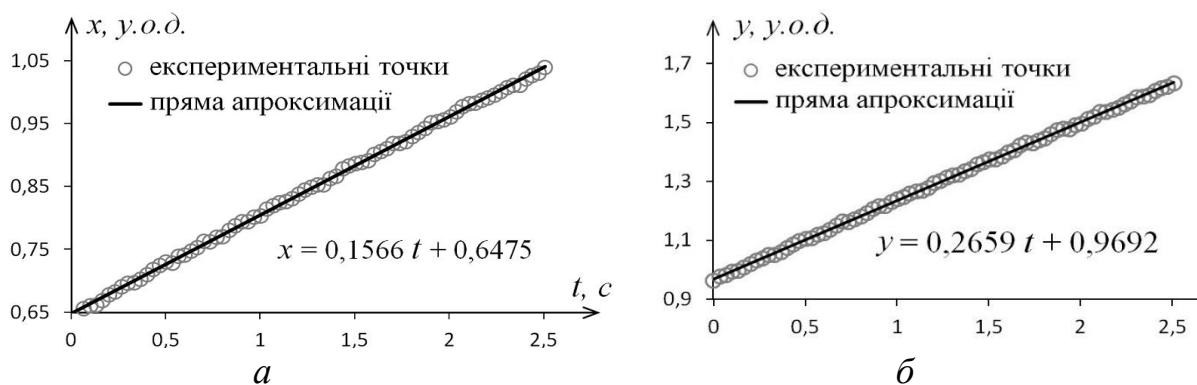
Рис. 3. Рівняння руху кульки за інерцією у невагомості.
